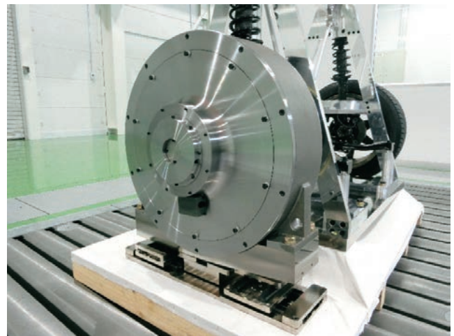
■ 扁平型ダイナモ外観(参考出展)
