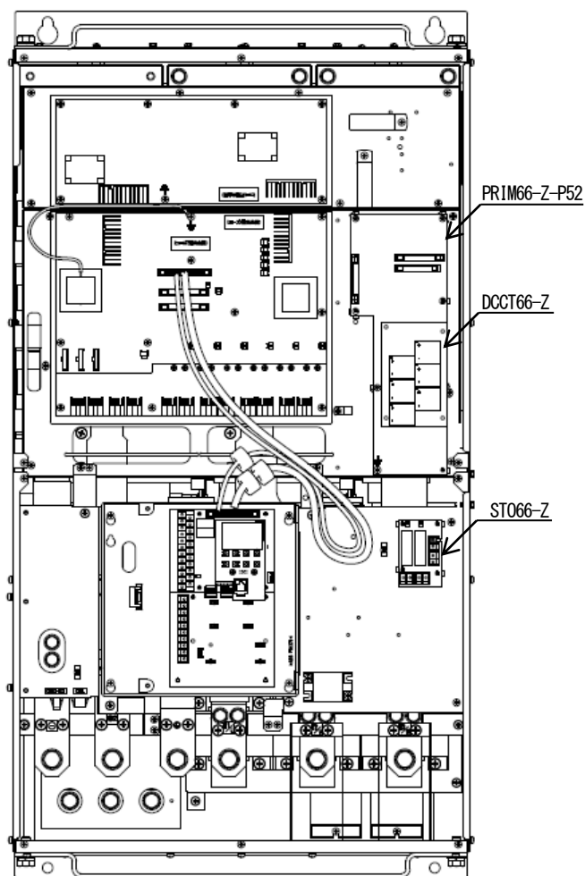
マスタ側 (型式:W52M)
