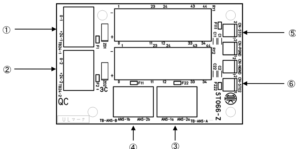
<ST066-Z>基板
