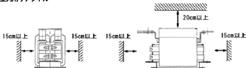
並列用リアクトル
