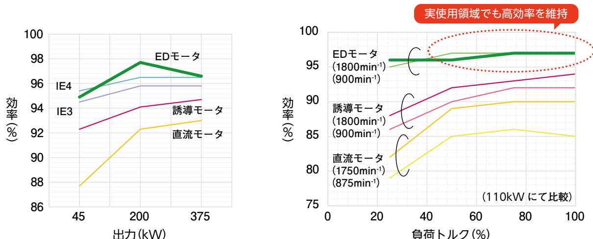
[出力・効率比較(100%負荷時)]
